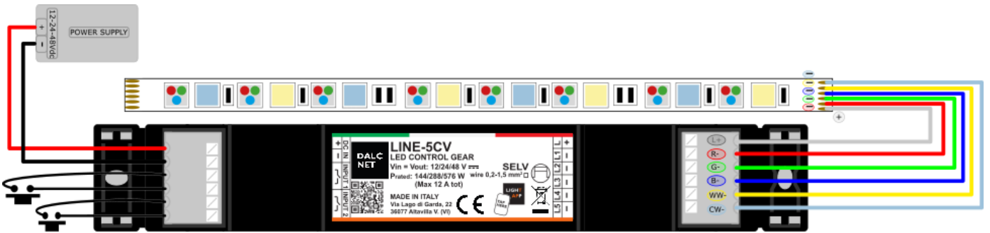
Figura 6: Schema di collegamento per carico LED RGB+TW
