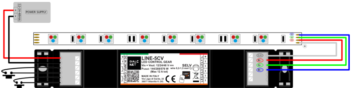
Figura 4: Schema di collegamento per carico RGB
