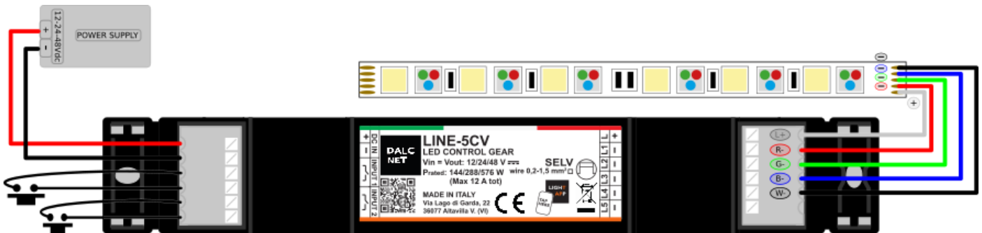
Figura 5: Schema di collegamento per carico LED RGBW
