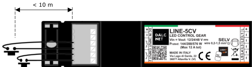
Figura 7: Collegamento del Comando Locale per brevi distanze
