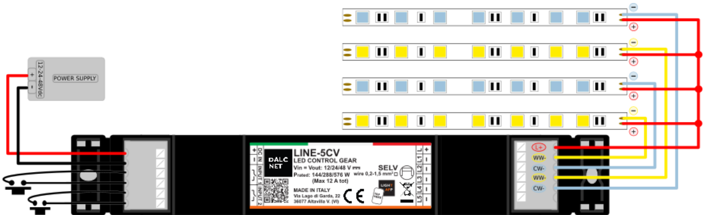
Figura 3: Schema di collegamento per carichi LED Bianco-Dinamico
